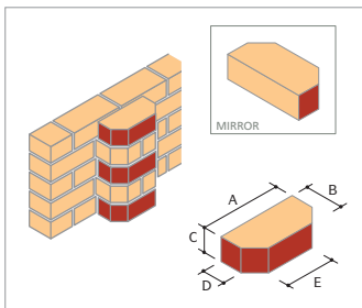
AN.6 Double Cant
