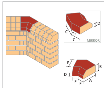
AN.11 Single Cant Internal Angle
