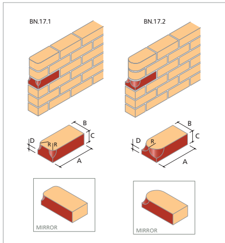
BN.17 Cownose Stop
