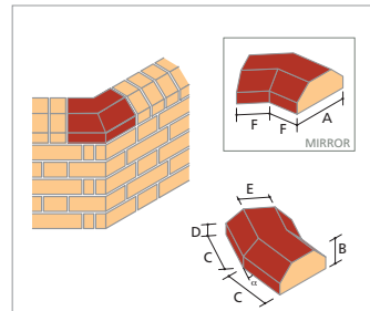
AN.18 Double Cant Angle
