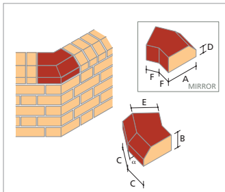
AN.10 Single Cant External Angle
